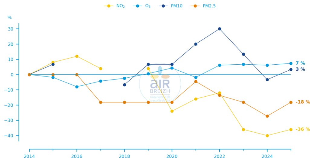
ÉVOLUTION DES PRINCIPAUX POLLUANTS RÉGLEMENTÉS DEPUIS 2014 (MOYENNES ANNUELLES) AUX STATIONS D'ILLE-ET-VILAINE
