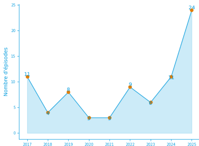
BILAN DES ÉPISODES DE POLLUTION DEPUIS 2017 (NOMBRE DE JOURS DE DÉPASSEMENT DE SEUIL EN ILLE-ET-VILAINE)
