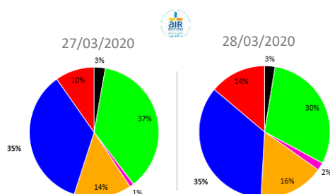
Composition chimique des PM1 à Rennes les 27 et 28 mars 2020
