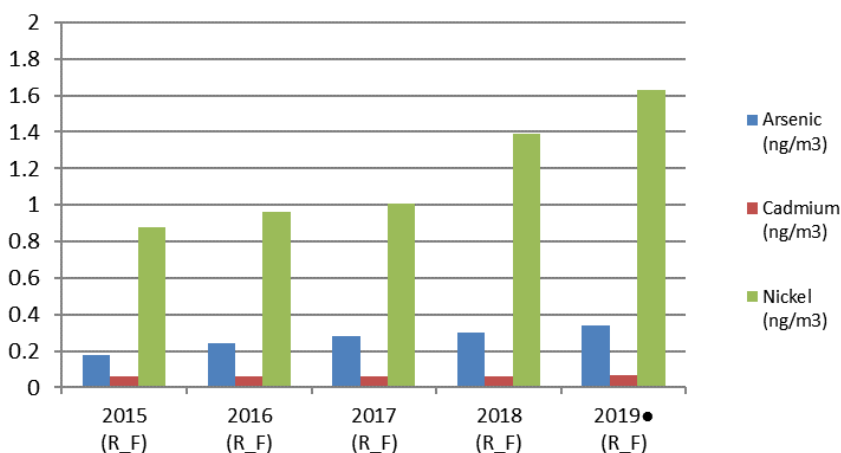
Evolution des concentrations moyennes annuelles en Arsenic, Cadmium et Nickel mesurées à Guipry (ng/m 3 )
