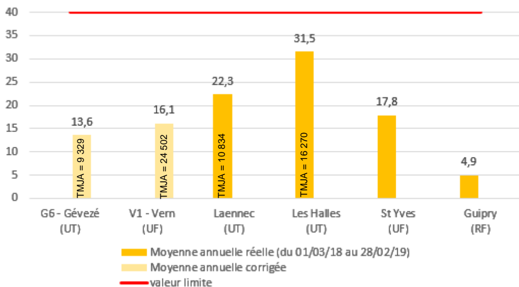
Figure 35 : Moyennes annuelles en dioxyde d'azote estimées et mesurées ('réelles')
