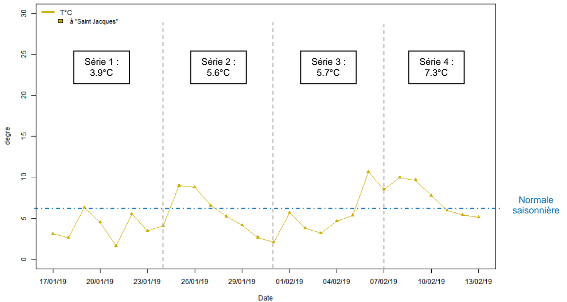
Figure 13 : Evolution des températures moyennes journalières en °C durant la campagne hivernale (station Météo France de St Jacques de la Lande)
