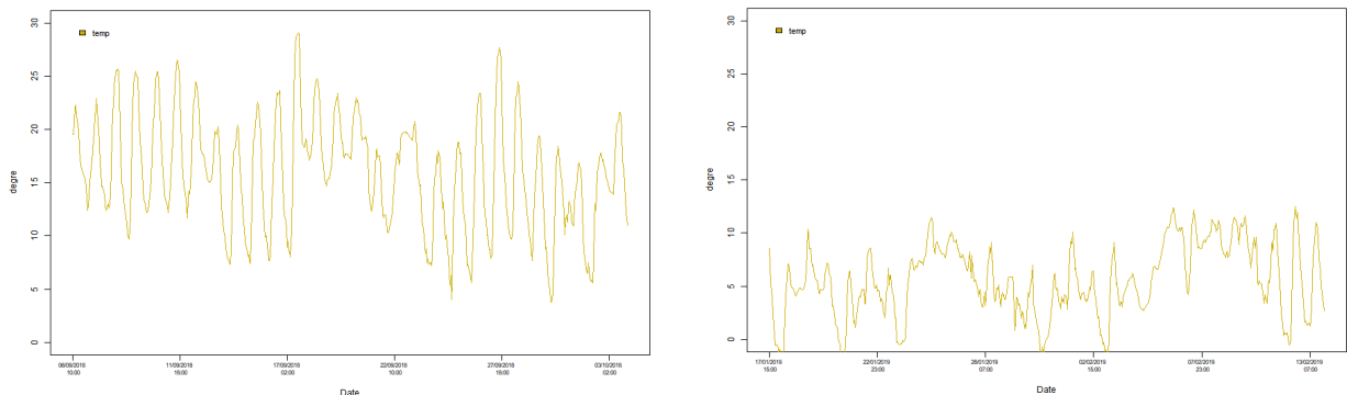
Figure 14 : Evolution horaire des températures en campagne estivale (à gauche) et hivernale (à droite) (station Météo France de St Jacques de la Lande)
