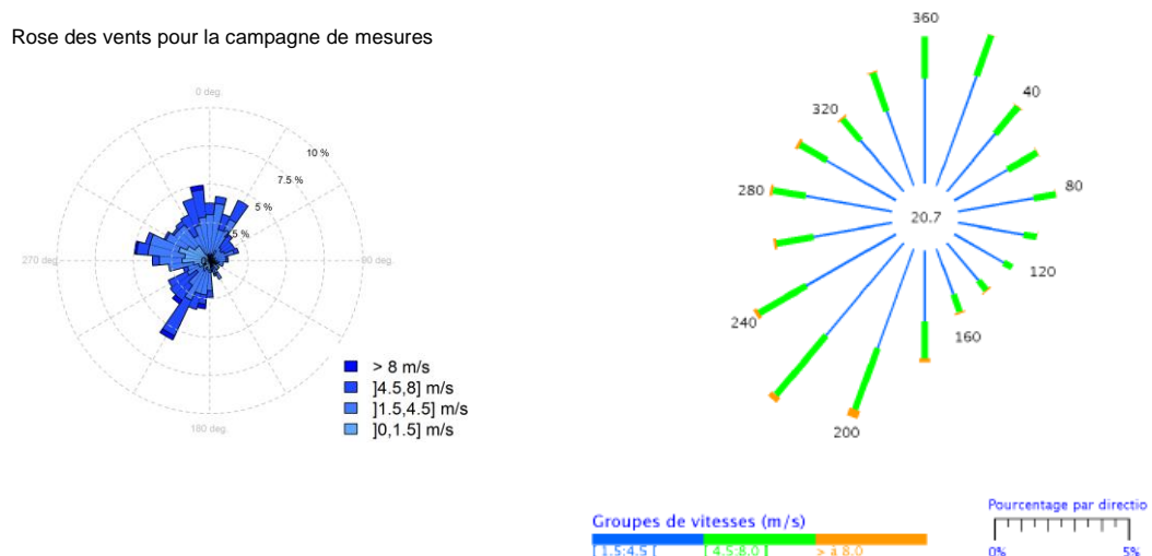
Figure 6 : Rose des vents durant la campagne de mesures estivale (à gauche) et rose des vents type d'un mois de septembre [données MF ST Jacques] (à droite)
