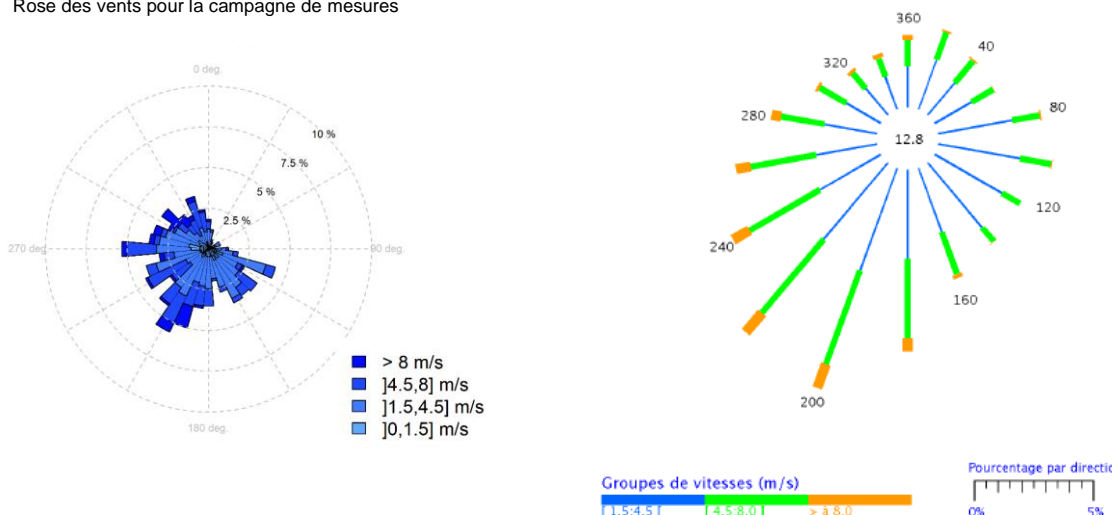
Figure 8 : Rose des vents durant la campagne de mesures hivernale (à gauche) et rose des vents type d'un mois de janvier [données MF ST Jacques] (à droite)
