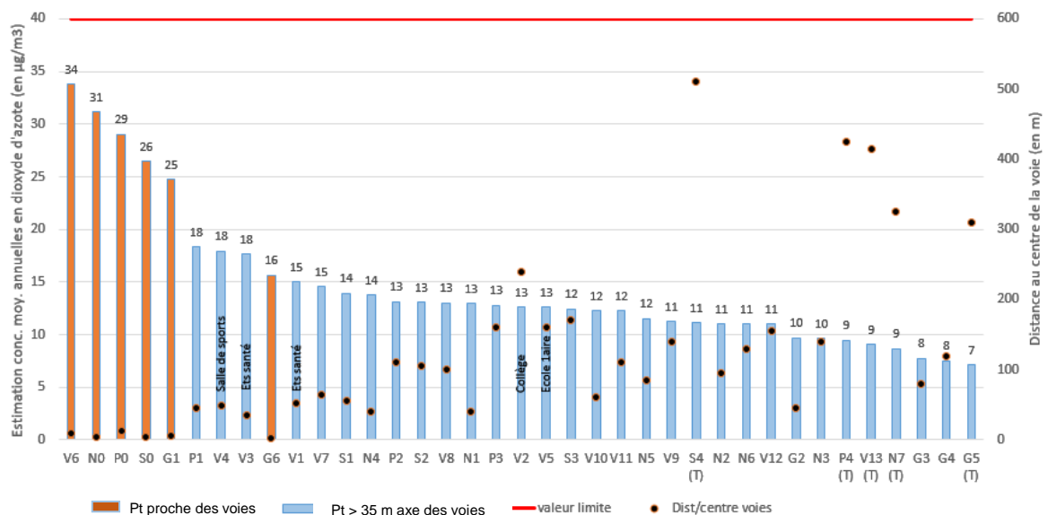
Figure 33 : Estimation des moyennes annuelles en dioxyde d'azote (axe de gauche en \mu\text{g}/\text{m}^3 ) et indication des distances par rapport à la voie de circulation (axe de droite en m)
