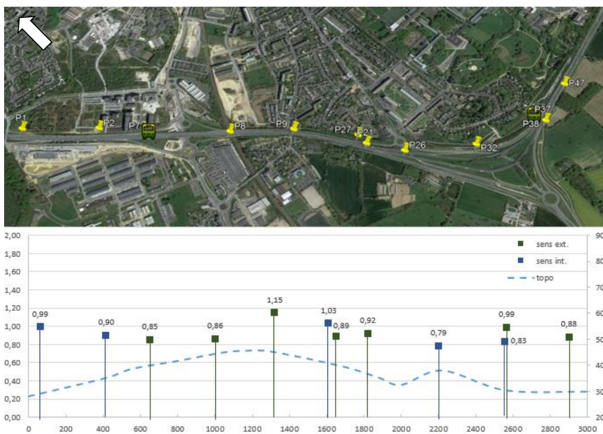
Figure 70 : Concentrations moyennes en benzène au bord de la rocade (axe de gauche, en \mu\text{g}/\text{m}^3 ) et topographie (axe de droite, en m)
