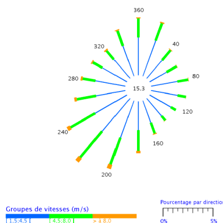
Normales des roses des vents sur l'année 1981 et 2010
