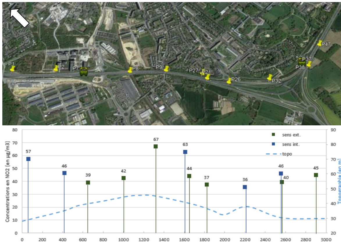
Figure 67 : Concentrations moyennes en dioxyde d'azote au bord de la rocade et topographie
