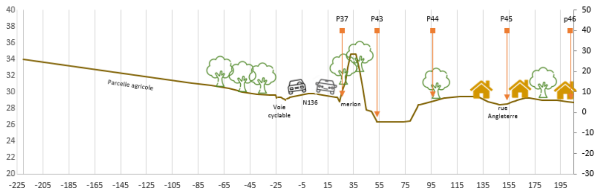
Figure 32 : Profil topographique (en m) – transect 7
