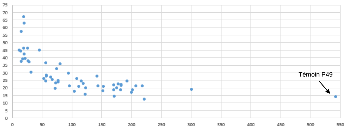
Figure 64 : Corrélation des niveaux de dioxyde d'azote (en \mu\text{g}/\text{m}^3 ) avec la distance des points (en m) par rapport à la rocade (centre des voies)
