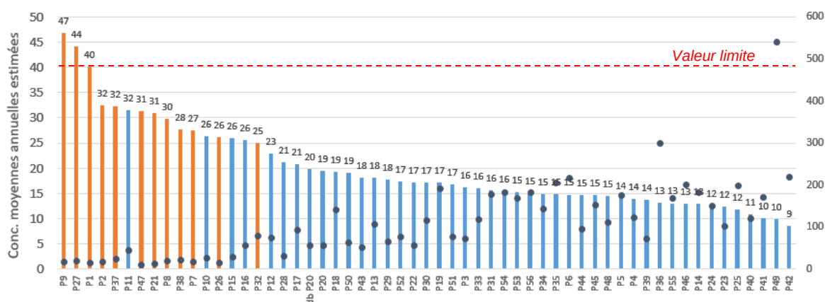
Figure 78 : Estimation des moyennes annuelles en dioxyde d'azote (axe de gauche en \mu\text{g}/\text{m}^3 ) et indication des distances par rapport à la voie de circulation (axe de droite en m)
