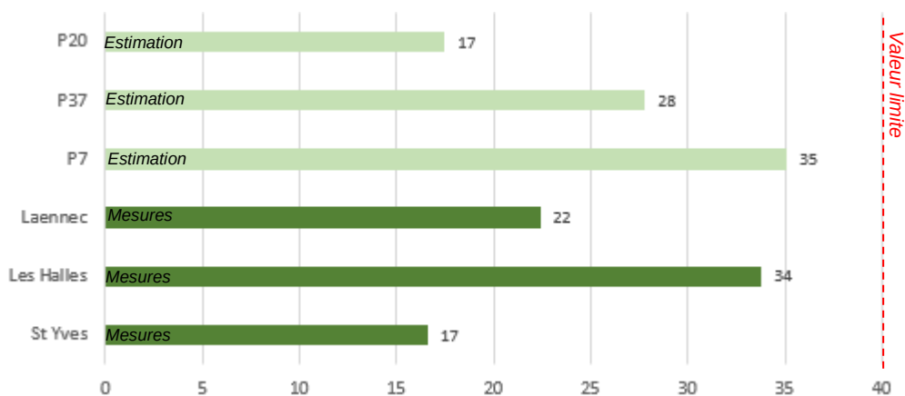
Figure 80 : Moyennes annuelles estimées et mesurées en dioxyde d'azote (du 01/11/17 au 30/10/18)
