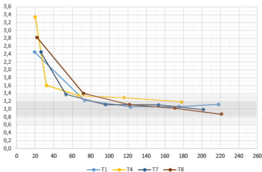
Figure 74 : Comparaison des profils de décroissances des rapports « concentrations dioxyde d'azote/niveau de fond » en fonction de l'éloignement des axes routiers (en m)
