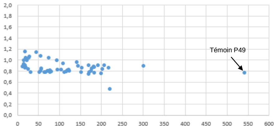
Figure 66 : Corrélation des niveaux de benzène (en \mu\text{g}/\text{m}^3 ) avec la distance des points (en m) par rapport à la rocade (centre des voies)
